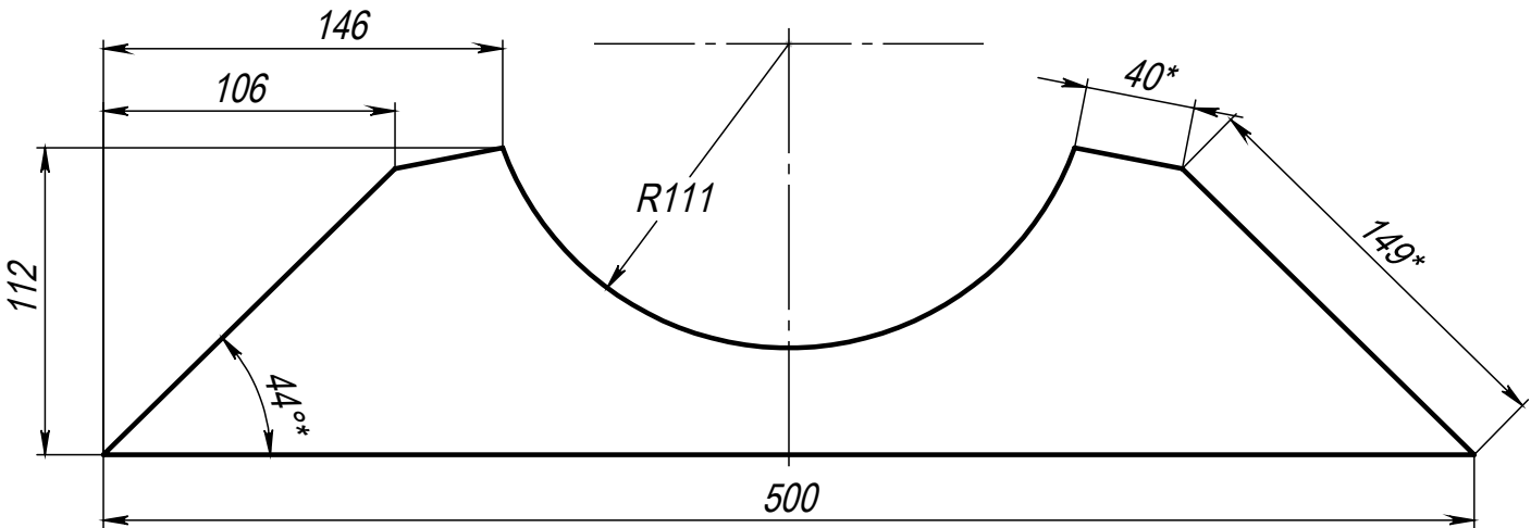
25.SHT.G.01.00.00.05 Пластина 2 шт.
