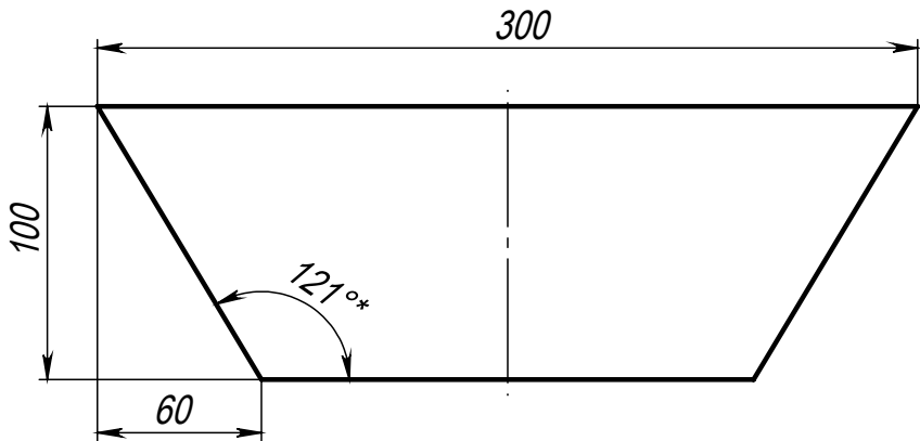
25.SHT.G.06.01.00.03 Пластина горловины 4 шт.
